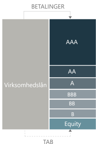
Figur 1. CLO-struktur stiliseret
